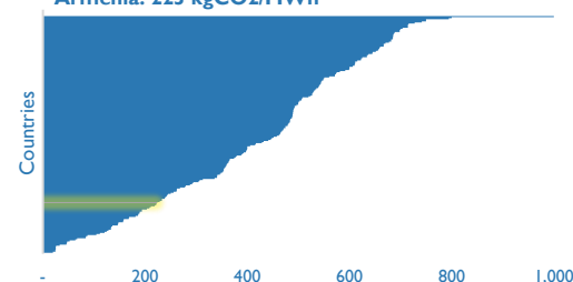
Armenia: 223 kgCO 2 /MWh
